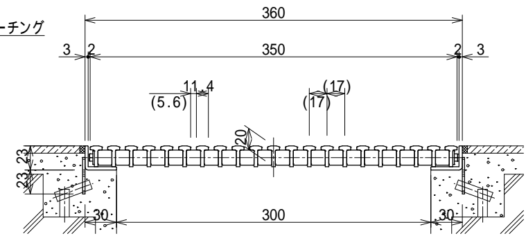
断面詳細図 S = 1 : 5
