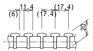
断面詳細 S = 1 : 3
