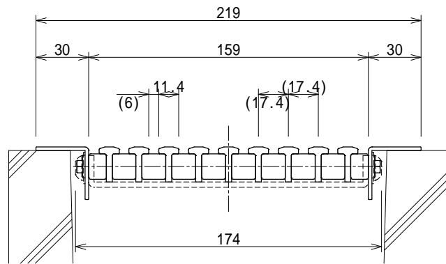
断面詳細図 S=1:3
