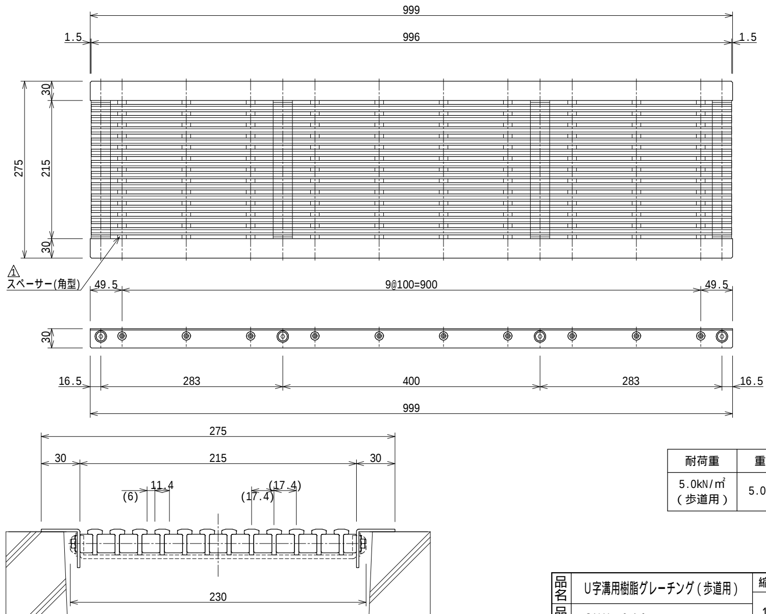
断面詳細図 S=1:3
