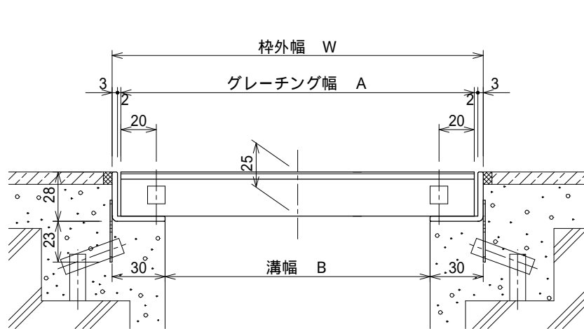
断面詳細図 S=1:3
