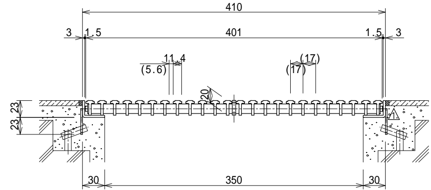
断面詳細図 S = 1 : 5
