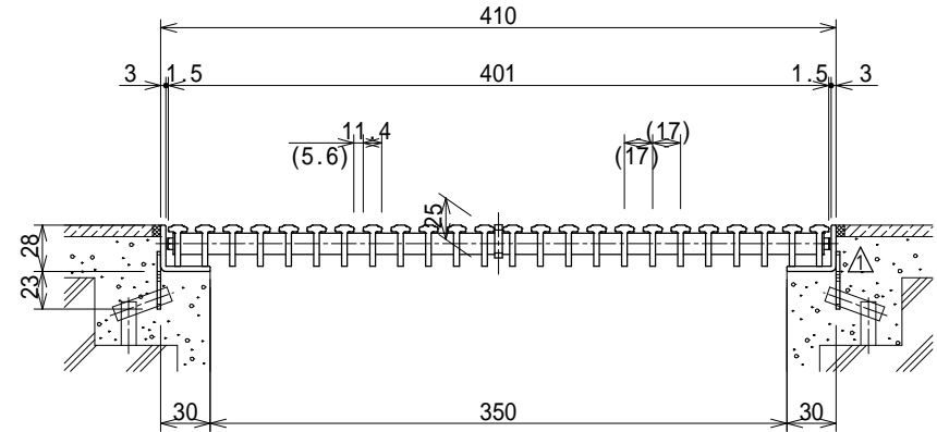
断面詳細図 S=1:5
