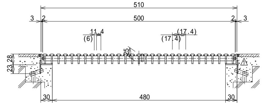
断面詳細図 S=1:6
