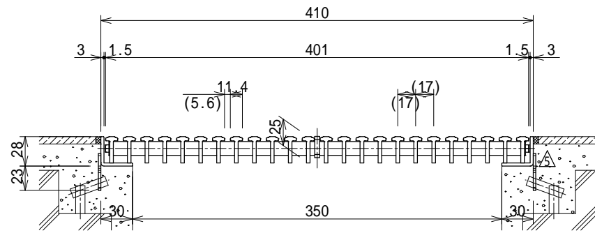
断面詳細図 S=1:5
