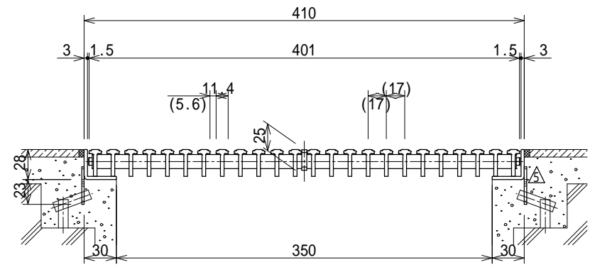
断面詳細図 S=1:5
