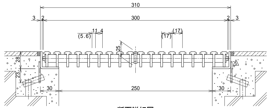
断面詳細図 S=1:3
