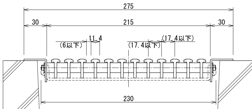
断面図 S=1:3
