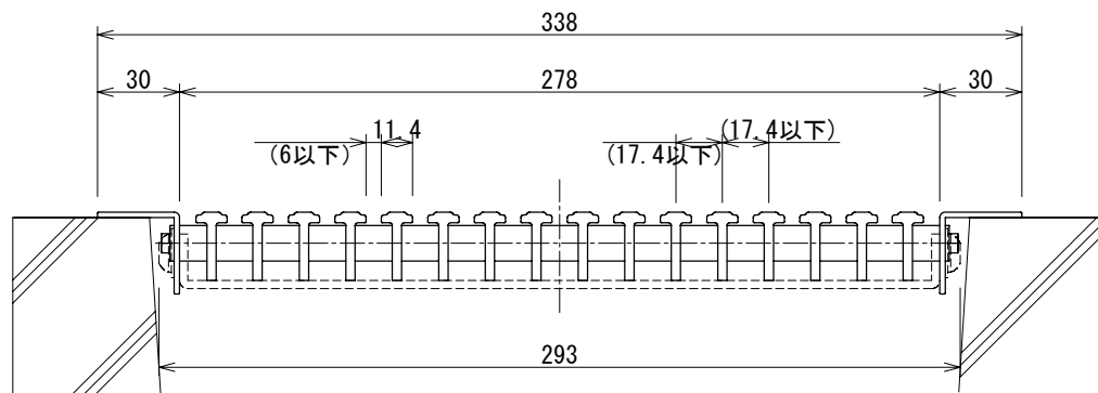
断面図 S=1:3
