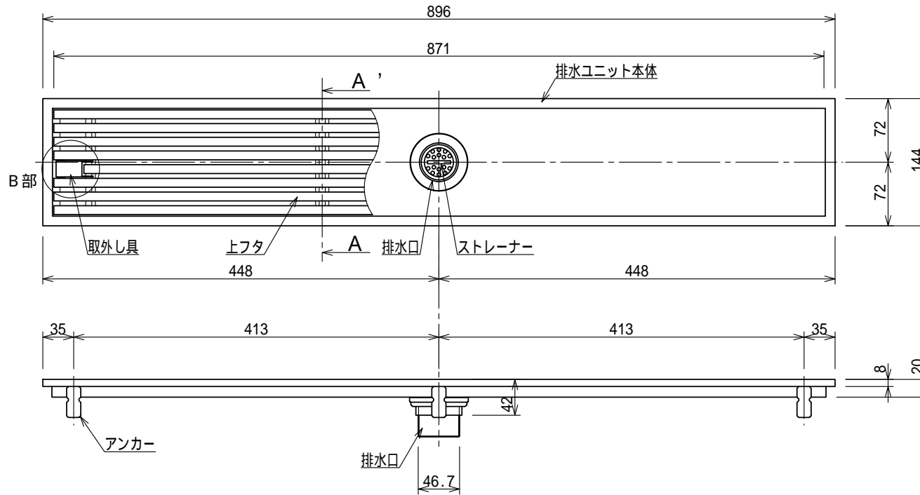
排水部詳細図 S=1:2
