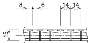
側面詳細 S = 1 : 3
