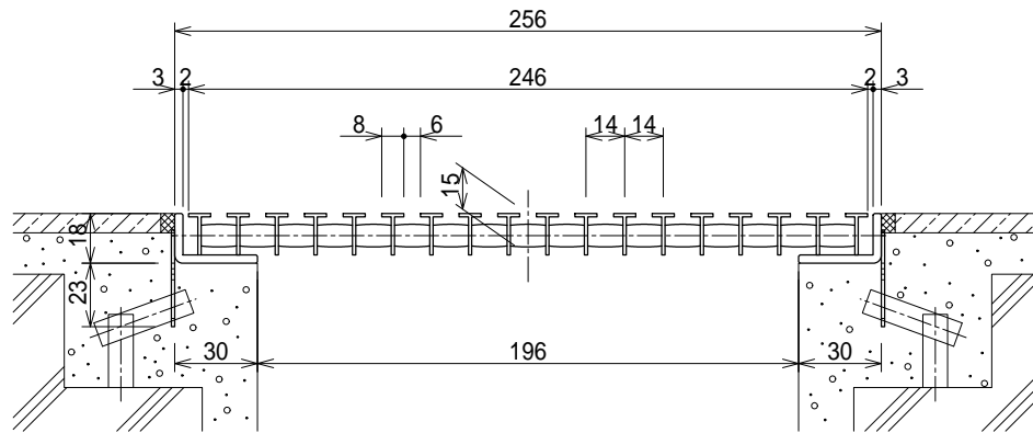
断面詳細図 S=1:3
