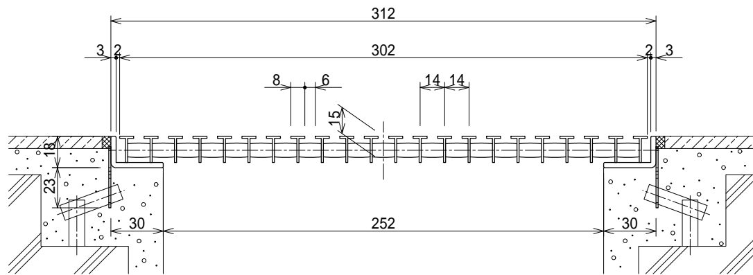
断面詳細図 S=1:3
