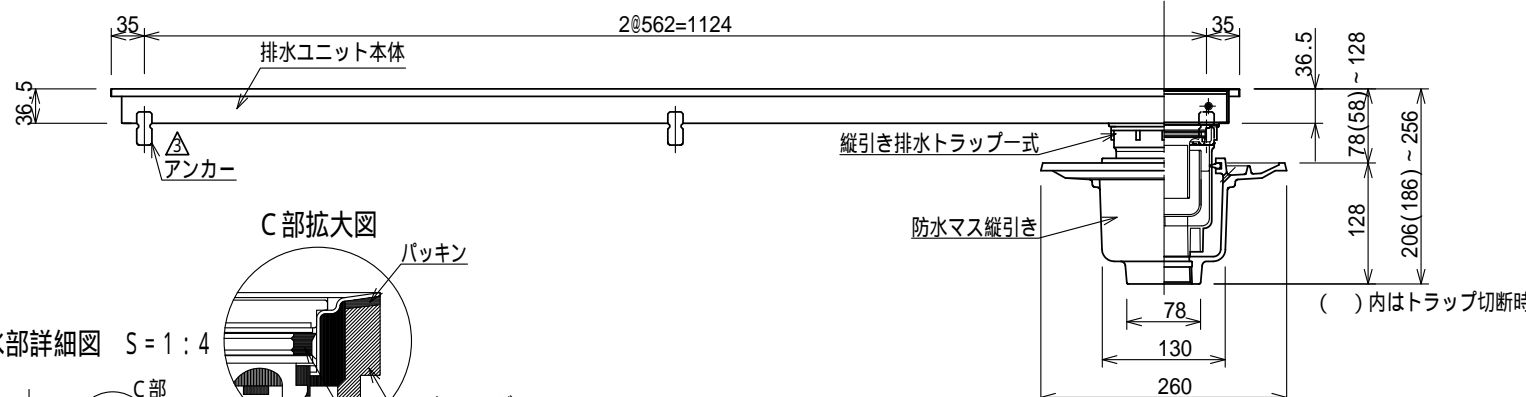
A - A' 断面図 S = 1 : 3
