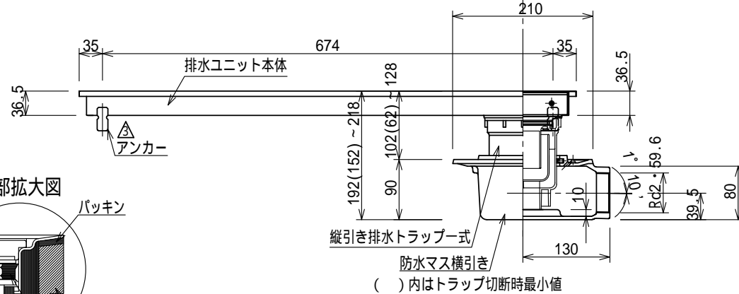
A - A' 断面図 S=1:3
