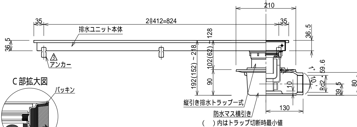
A - A' 断面図 S=1:3
