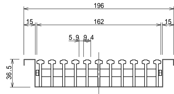
A - A' 断面図 S=1:3
