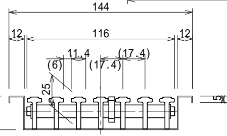
断面詳細図 S=1:3
