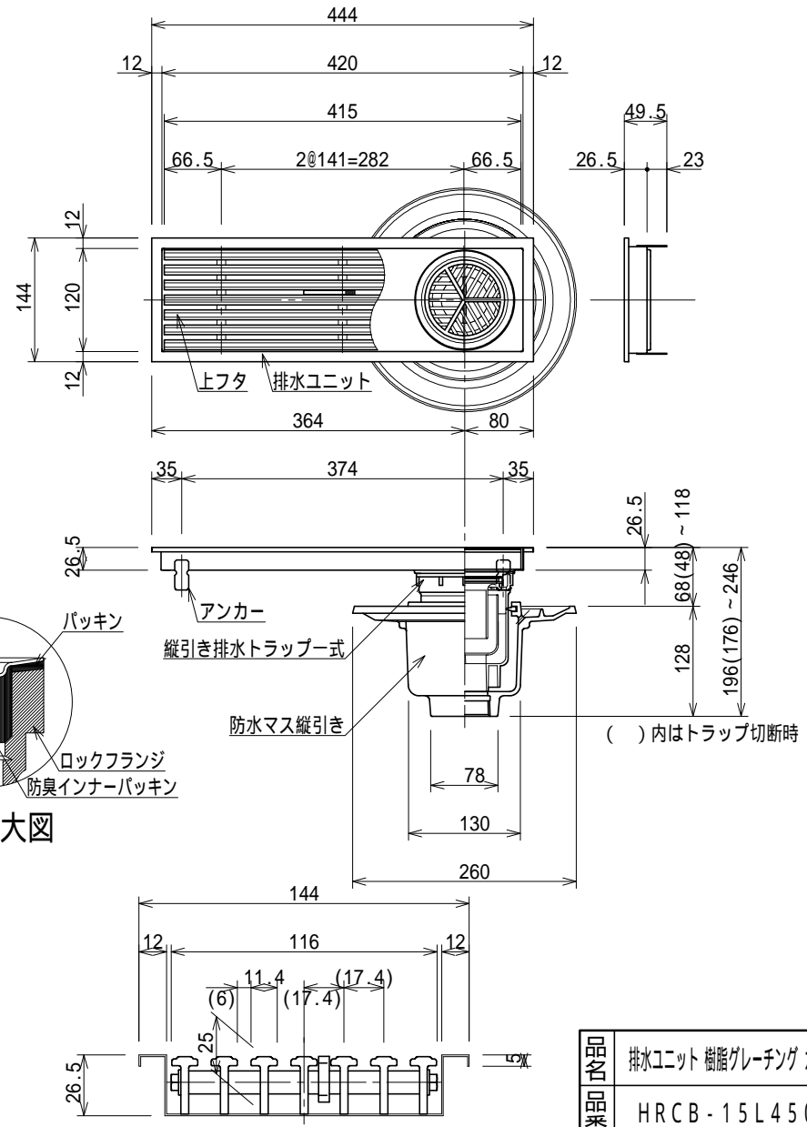
断面詳細図 S=1:3
