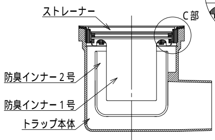
排水部詳細図 S=1:4
