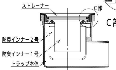
排水部詳細図 S=1:4
