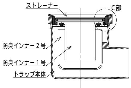
排水部詳細図 S=1:4
