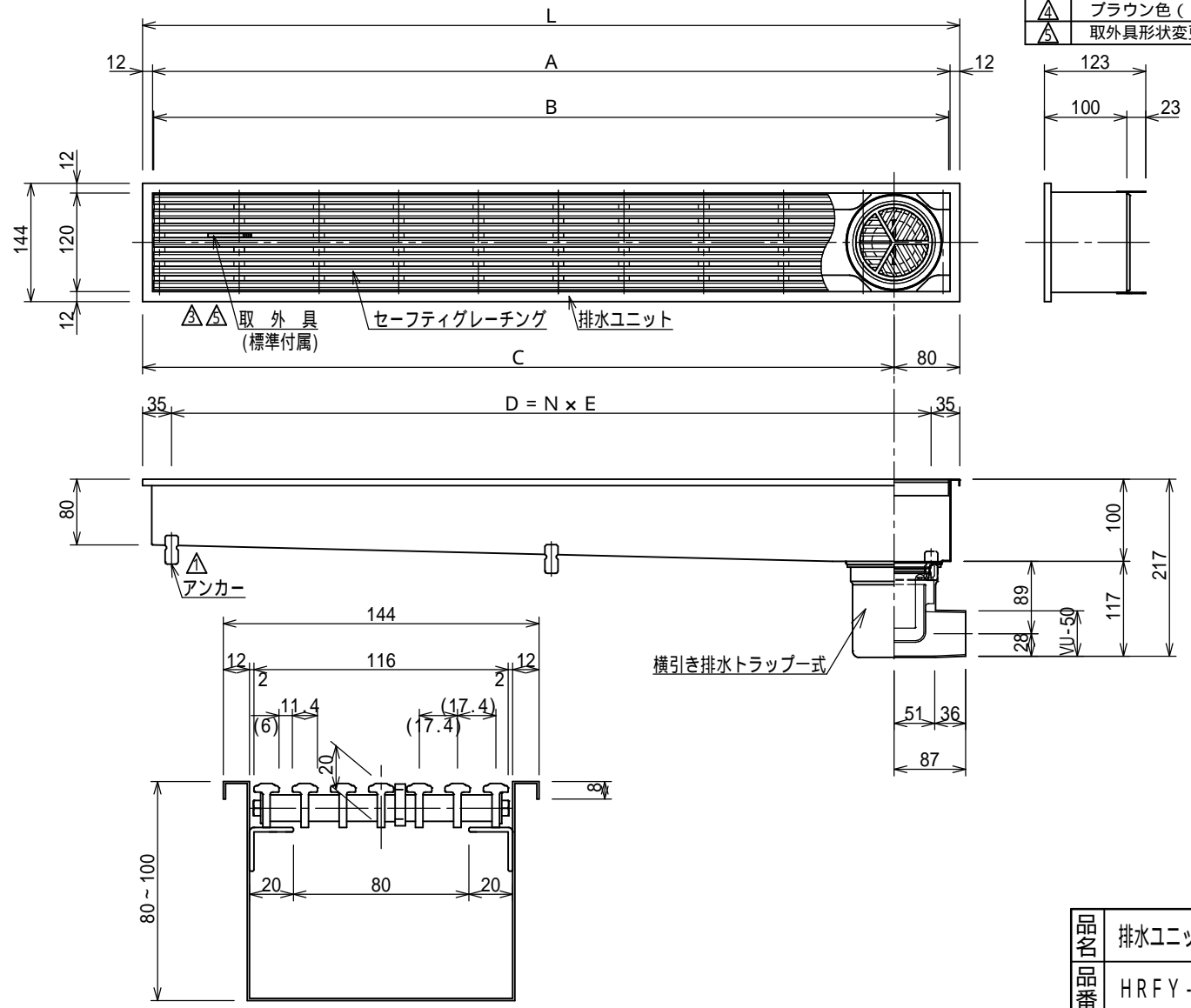
断面詳細図 S=1:3
