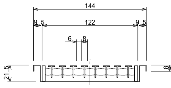
断面詳細図 S=1:3
