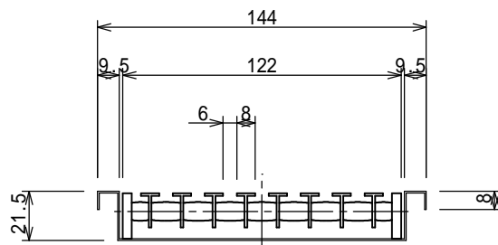
断面詳細図 S=1:3
