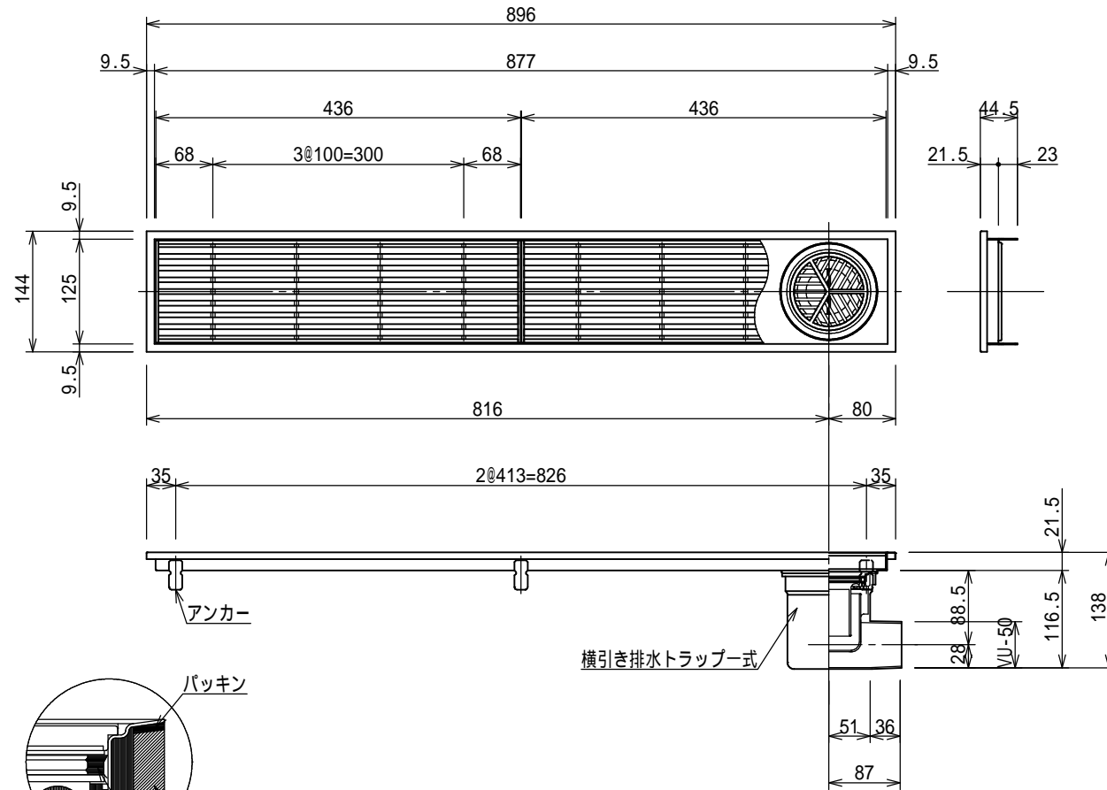
C部拡大図
