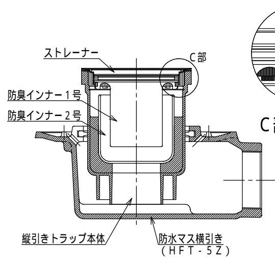
排水部詳細図 S=1:4
