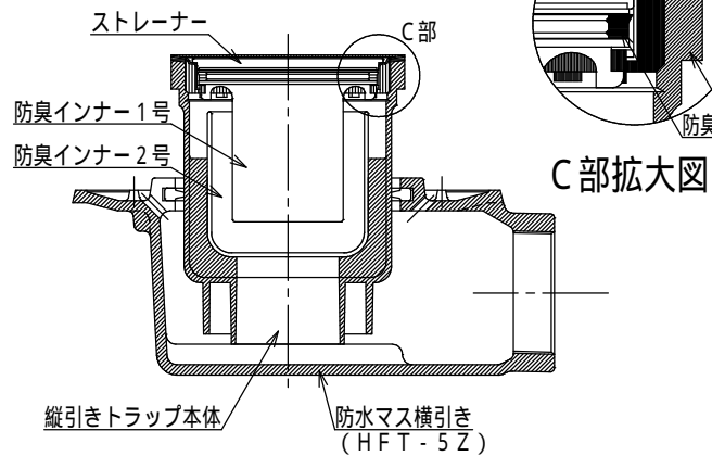
排水部詳細図 S=1:4
