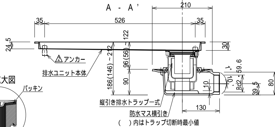
断面図
