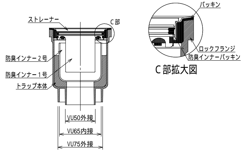
排水部詳細図 S=1:4
