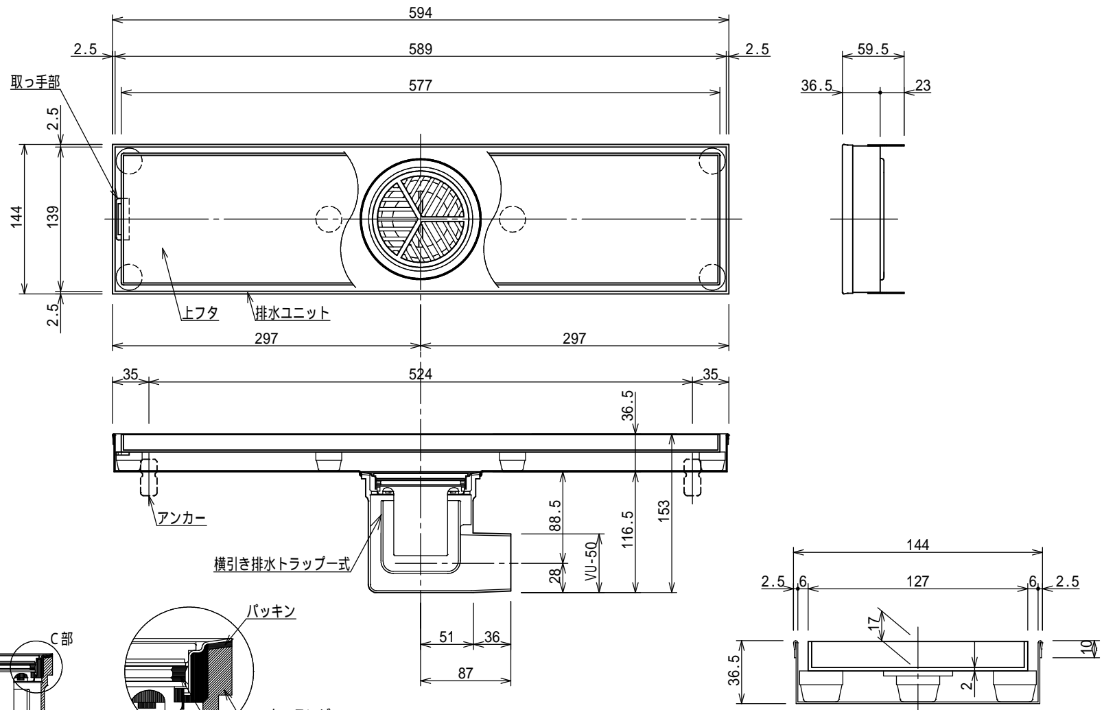
断面詳細図 S=1:3
