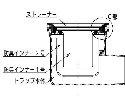
排水部詳細図 S=1:4
